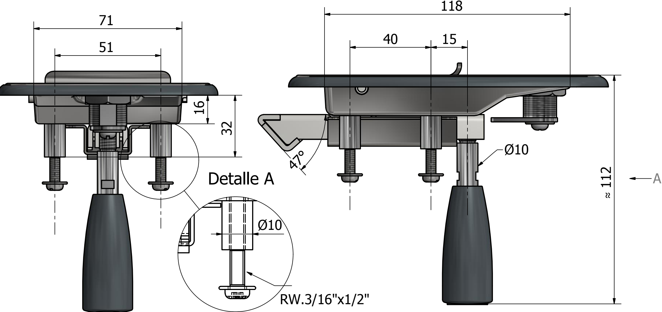
VISTA A
